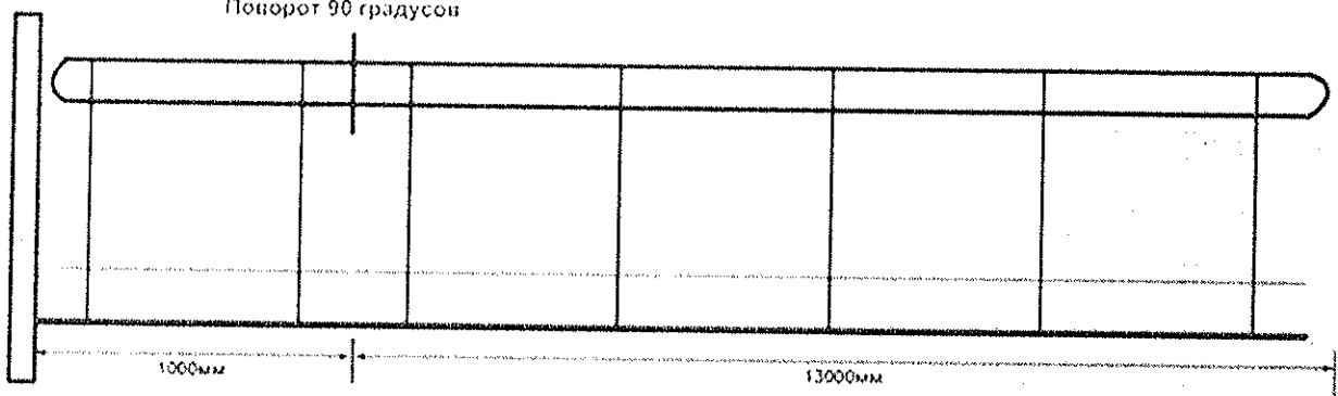
Вид сбоку
